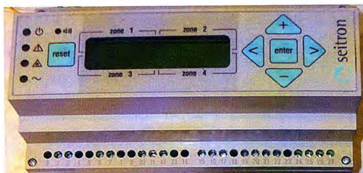
Рисунок 2 – Внешний вид блока RGY 000 MBP4
