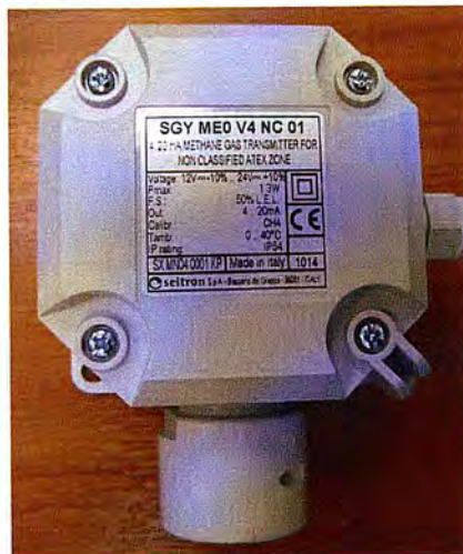
Рисунок 1 – Внешний вид сигнализаторов загазованности SGY, SGW
