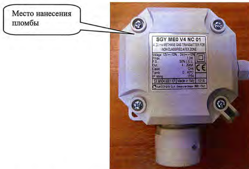
Рисунок 4 – Схема пломбирования сигнализаторов загазованности SGY, SGW
