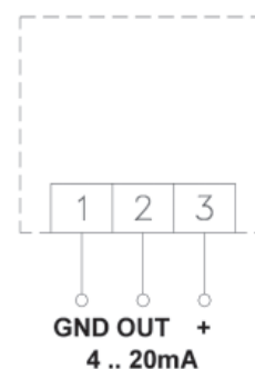
Рис. 5: Электрическое подсоединение
