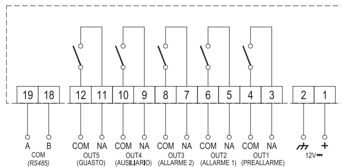
Рис. 1. Схема подключения
